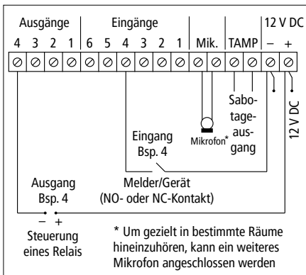
Anschluss-Diagramm
