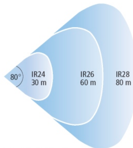
Infrarot-Ausleuchtungsfläche im Außenbereich (850 nm Strahler)
